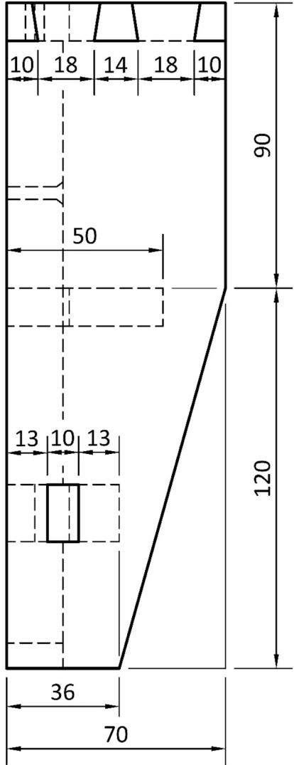
End View/Taobhchló
